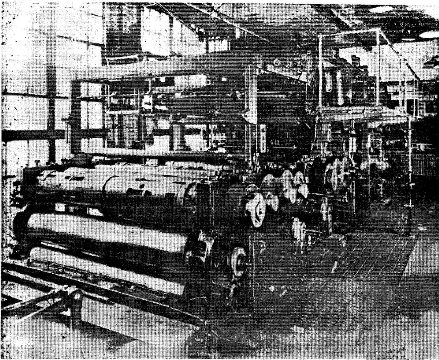
Foto de la Rotativa HOE instalada ya en los Talleres de "La Nación"
